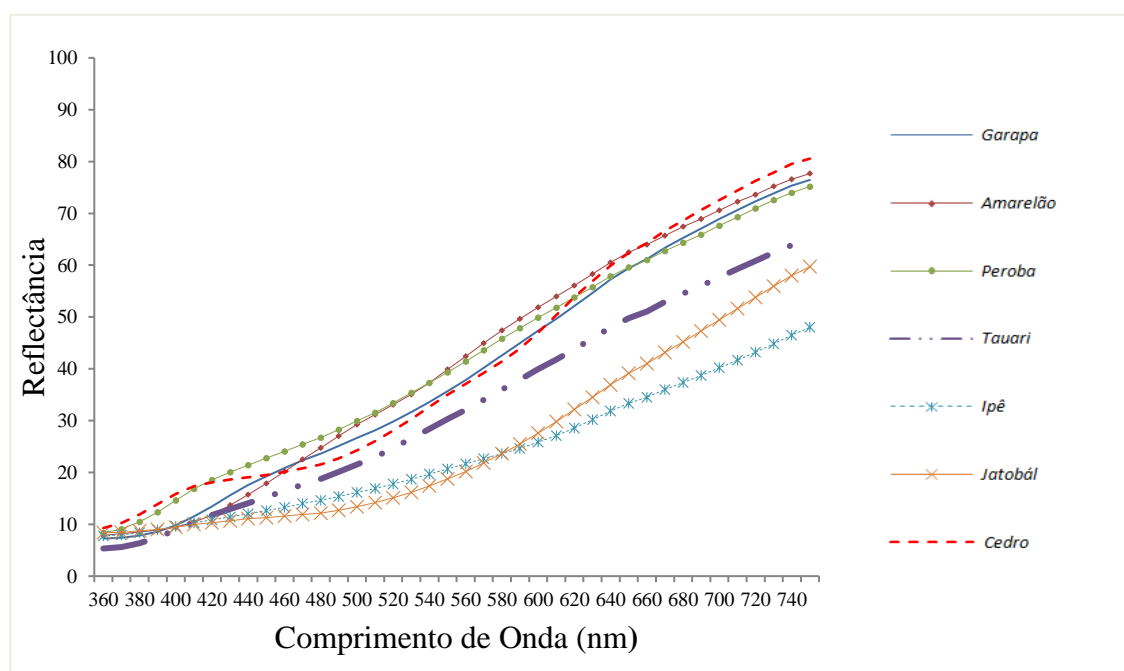
Figura 3. Assinatura espectral na região do visível de sete espécies florestais amazônicas.
