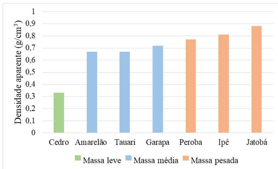
Figura 2. Valores médios de massa específica aparente das madeiras de espécies florestais amazônicas.
